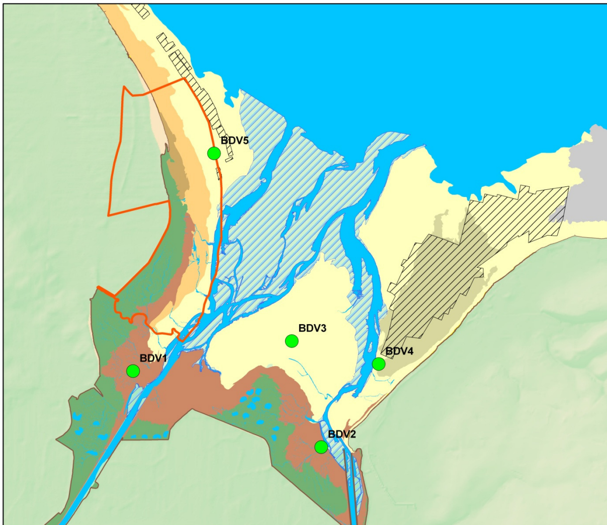
Evolution des principaux faciès biomorphosédimentaires de la baie des Veys. Points échantillonnés et complexes d'habitats Eunis.
